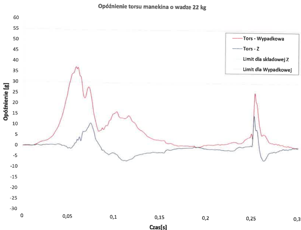
Wykres 2. Przebiegi opóźnień torsu manekina 22 kg podczas testu dynamicznego Graph 2. Decelerations of the chest for 22 kg dummy during dynamic test
