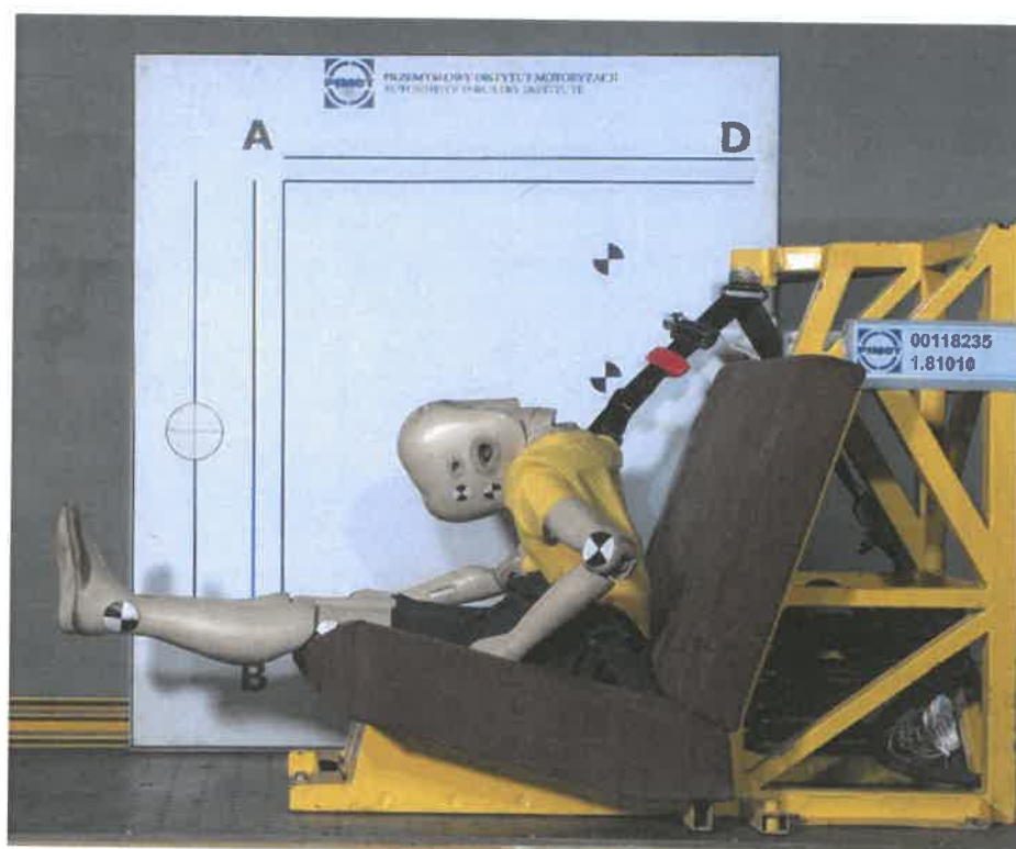
Fot. 3. Maksymalne przemieszczenie głowy manekina 32 kg podczas testu dynamicznego Pic. 3. Maximum displacement of the head 32 kg dummy during dynamic test
