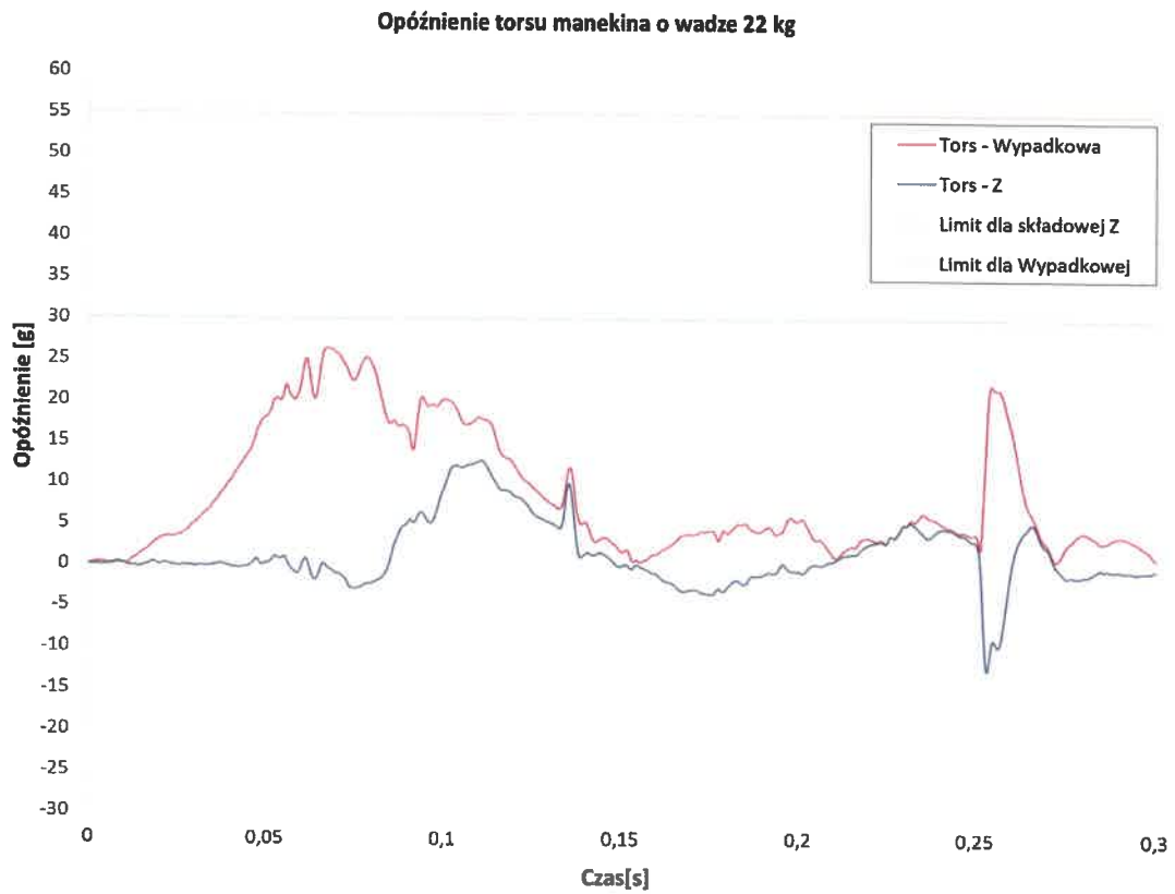
Wykres 3. Przebiegi opóźnień torsu manekina 22 kg podczas testu dynamicznego Graph 3. Decelerations of the chest for 22 kg dummy during dynamic test
